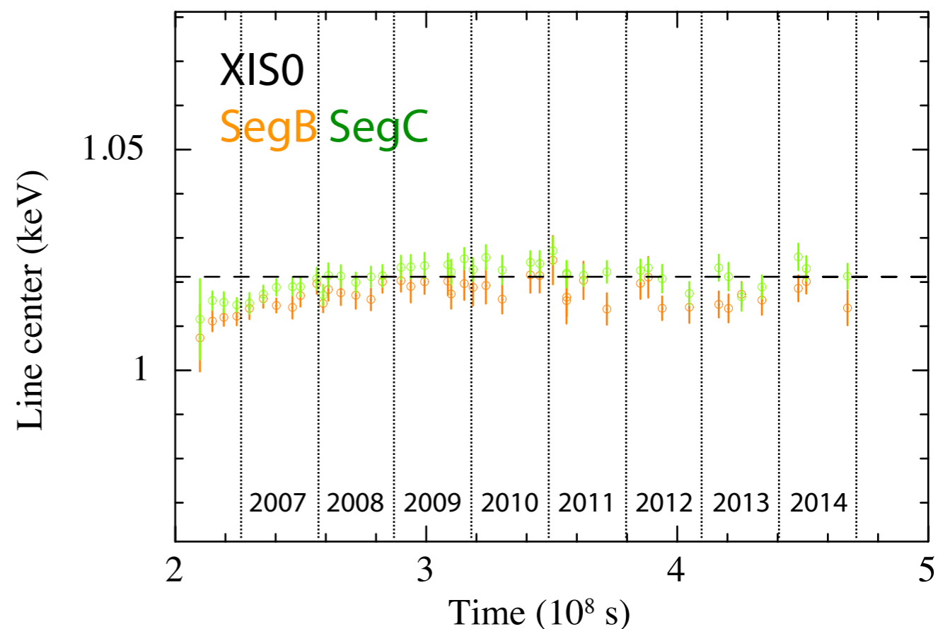
E0102 Ne x Lya (~1 keV)
