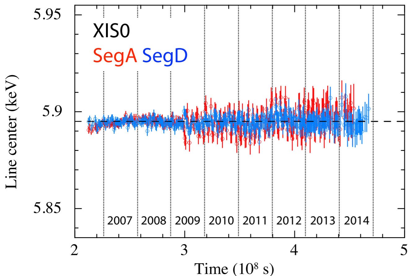
^{55}\text{Fe} Mn K \alpha (~6 keV)
