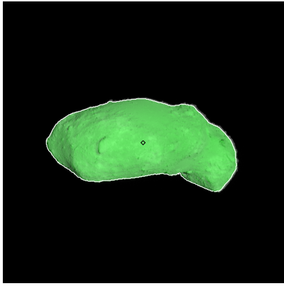
Figure 334: ST_2421134209_v.fits
