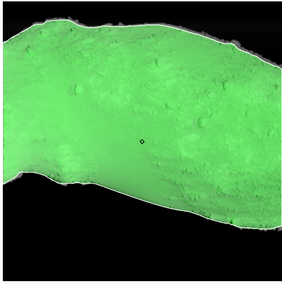
Figure 595: ST_2495748476_v.fits
